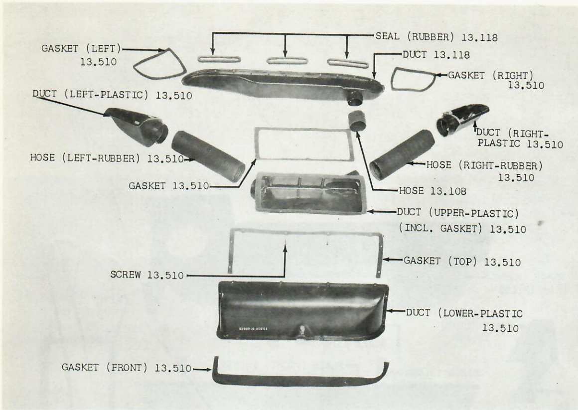
GROUP 13 - FIG. 4 - EVAPORATOR DUCTS 10-20-80 (WAC)
